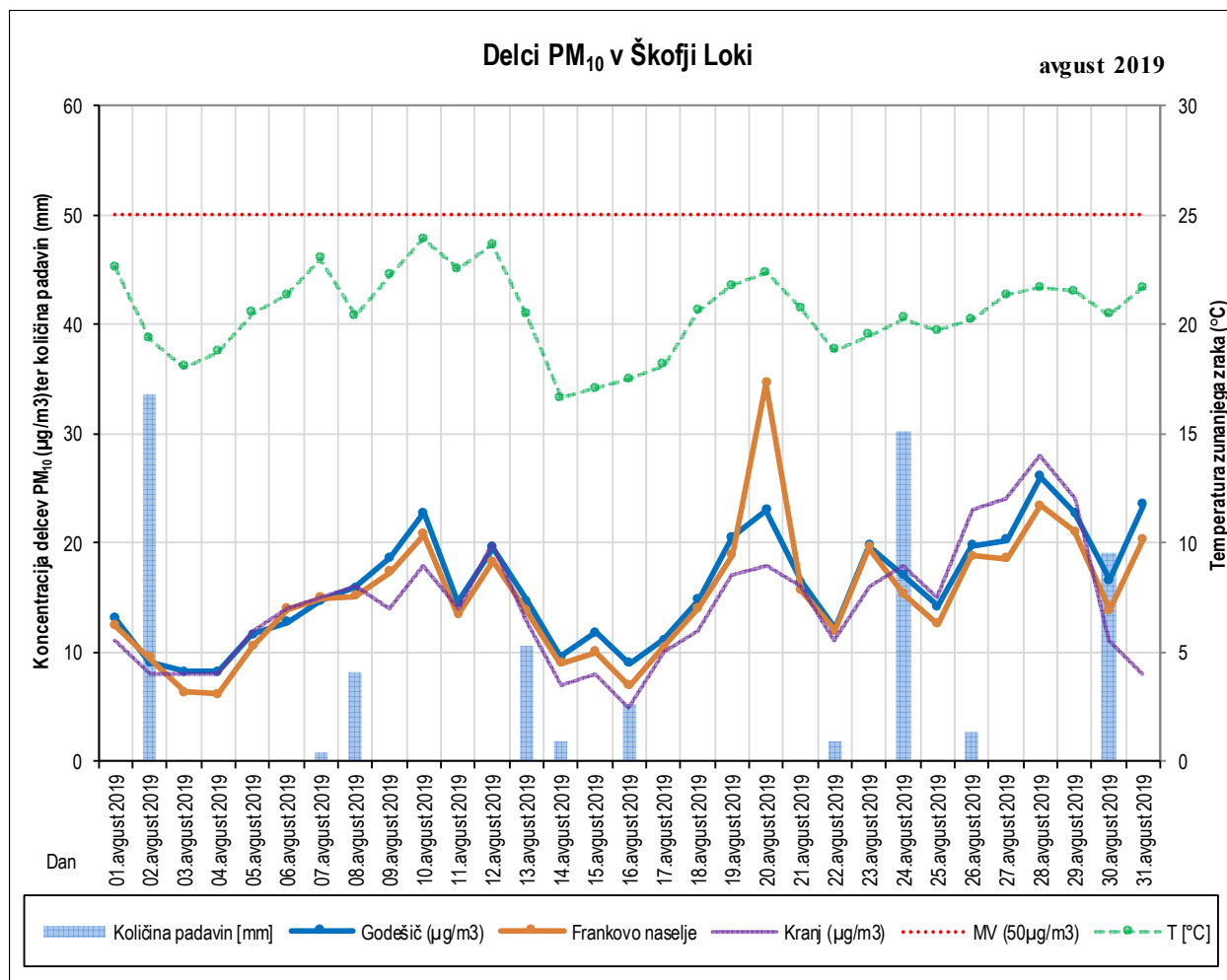
Slika 3: Potek izmerjenih dnevnih koncentracij delcev PM 10
